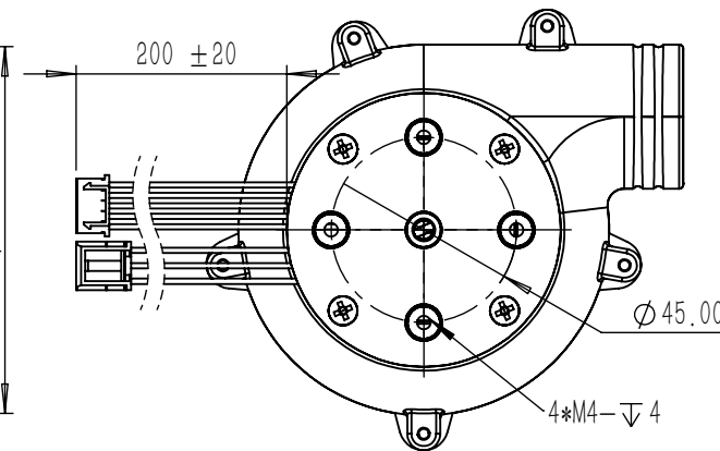
局部视图 C
